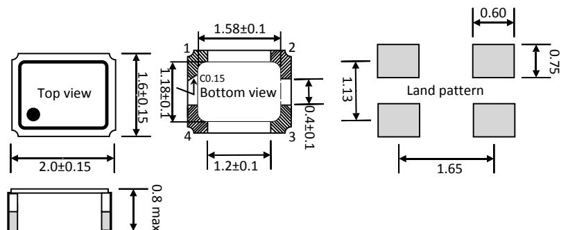
Dimensions(Unit:mm)
